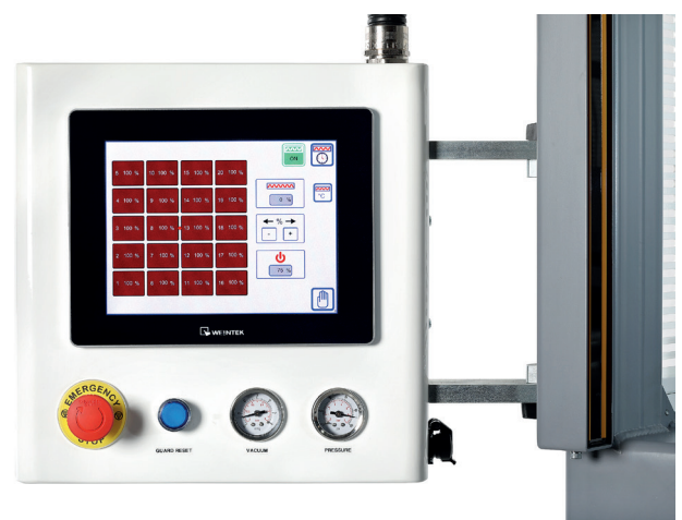
20 zones de chauffes contrôlables indépendamment (1 % de précision)
